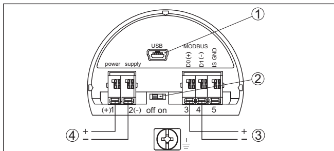
Abb. 6: Anschlussraum
