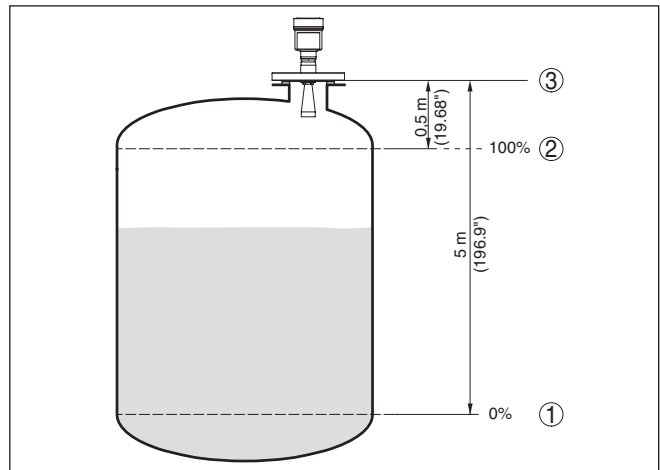
Abb. 8: Parametrierbeispiel Min.-/Max.-Abgleich
