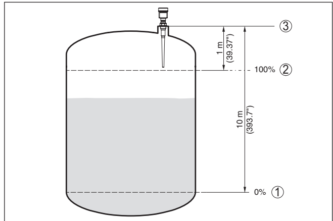
Abb. 8: Parametrierbeispiel
