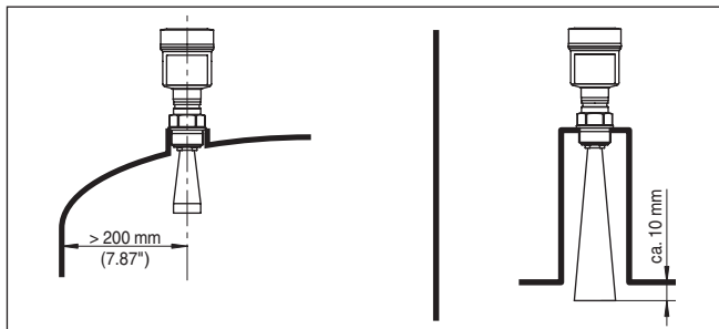
Abb. 2: Abstände der Antenne zu Behälterwand/Behälterdecke
