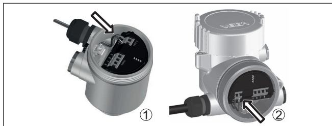
Abb. 3: Anschlusschritte 5 und 6
