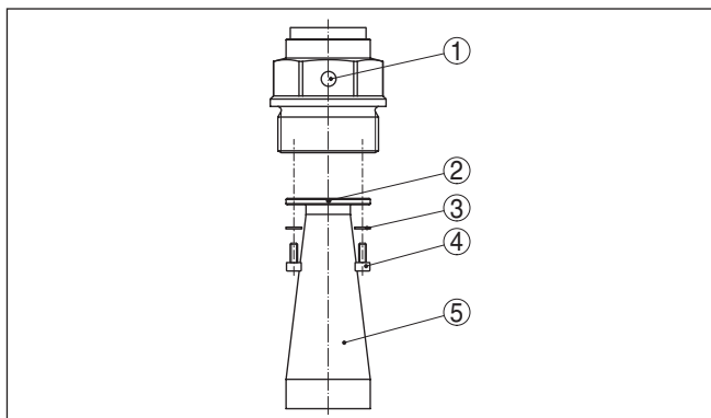
Fig. 3: Demontage hoornantenne
