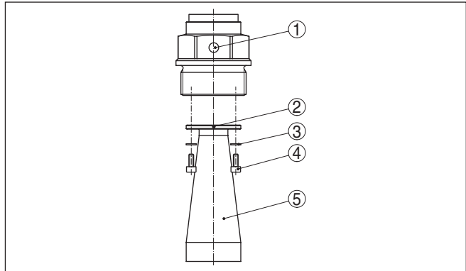
Fig. 3: Demontage hoornantenne
