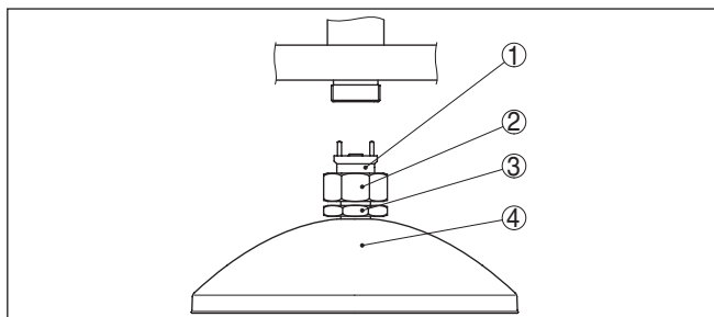
Fig. 2: Demontage paraboolantenne.
