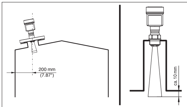
Fig. 5: Afstanden van de antenne tot de tankwand/tankdak
