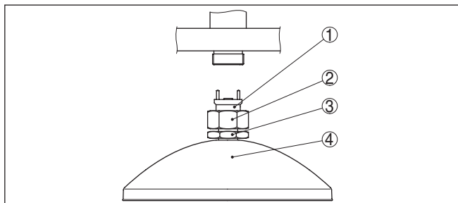
Fig. 4: Demontage paraboolantenne.
