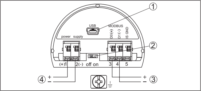
Fig. 9: Aansluitruimte
