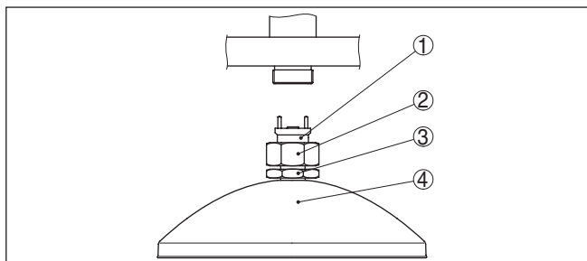
Fig. 2: Demontage paraboolantenne.
