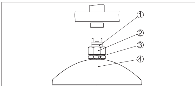
Fig. 4: Demontage paraboolantenne.
