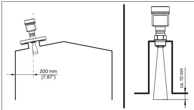
Abb. 5: Abstände der Antenne zu Behälterwand/Behälterdecke
