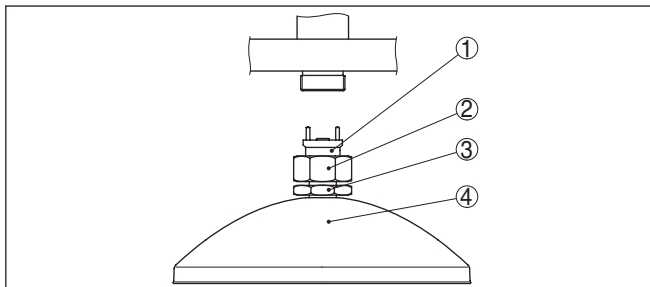
Abb. 2: Demontage Parabolantenne
