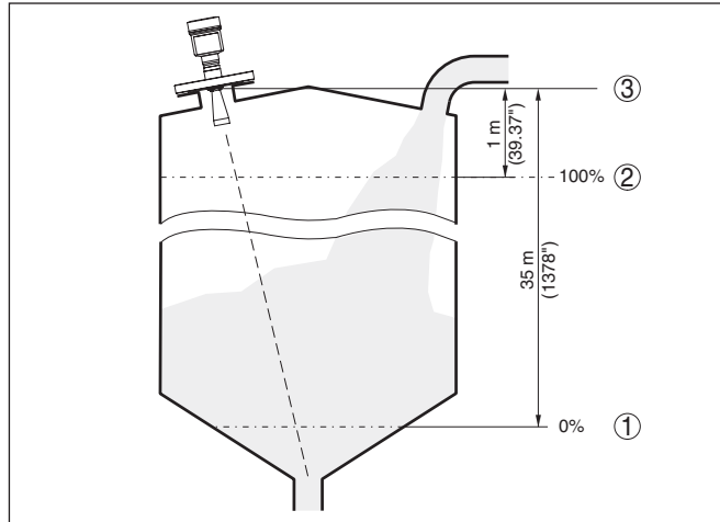
Abb. 11: Parametrierbeispiel
