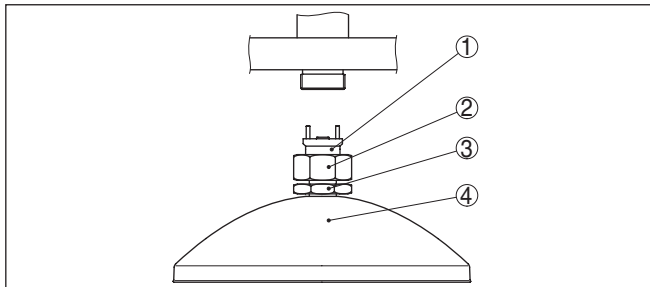
Abb. 4: Demontage Parabolantenne
