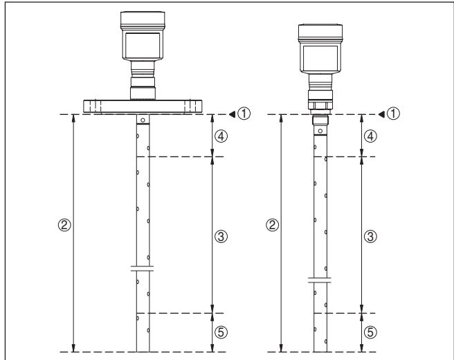
Abb. 8: Messbereiche - VEGAFLEX 81
