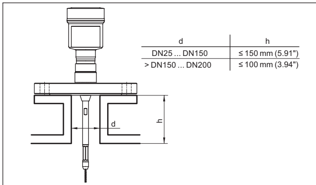
Abb. 4: Montagestutzen
