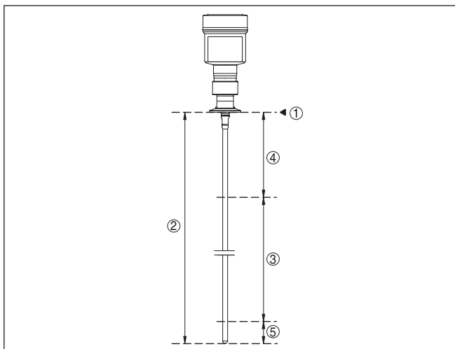
Abb. 11: Messbereiche - VEGAFLEX 83
