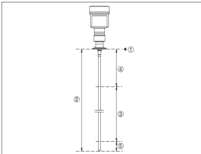
Fig. 11: Meetbereiken - VEGAFLEX 83
