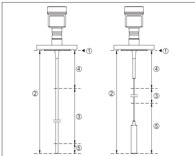
Abb. 11: Messbereiche - VEGAFLEX 83
