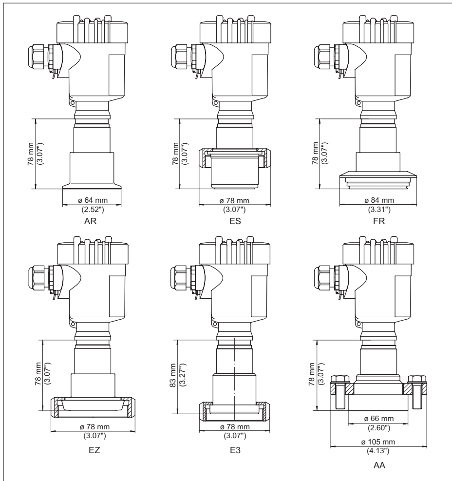
Rys. 41: VEGABAR 83, przyłącze higieniczne +150 °C (cela pomiarowa METEC®)
