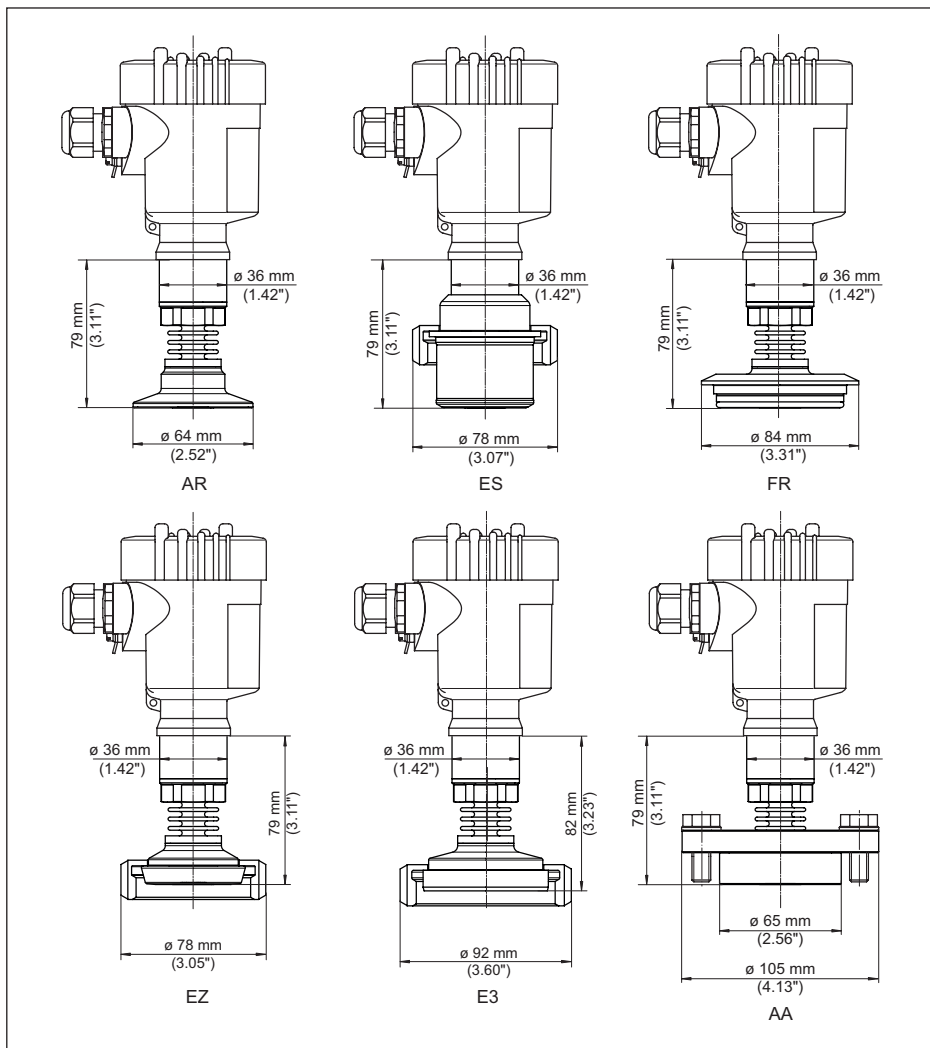
Rys. 40: VEGABAR 83, przyłącze higieniczne +150 °C (cela pomiarowa piezorezystancyjna/tensometryczna)
