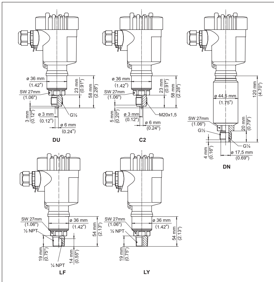
Rys. 37: VEGABAR 83, przyłącze gwintowane czołowo nie współpłaszczyznowe
