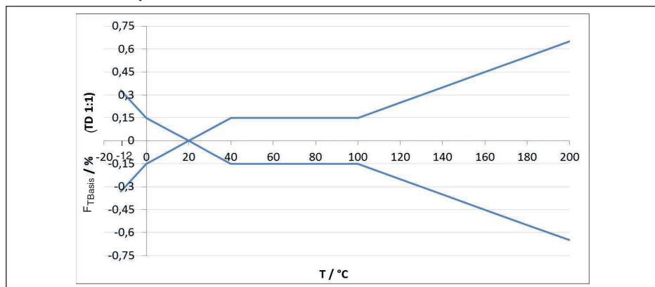
Rys. 27: Bazowy błąd temperatury F_{TBasis} przy TD 1 : 1
