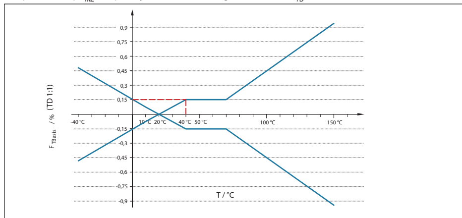
Rys. 33: Wyznaczenie bazowego błędu temperatury dla powyższego przykładu: F_{\text{TBasis}} = 0,15 %
