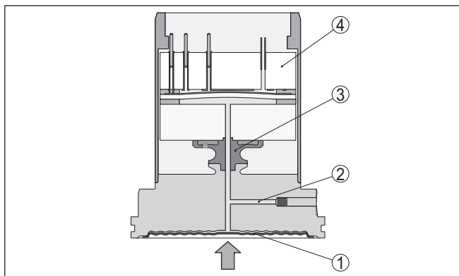
Rys. 4: Budowa celi pomiarowej METEC®
