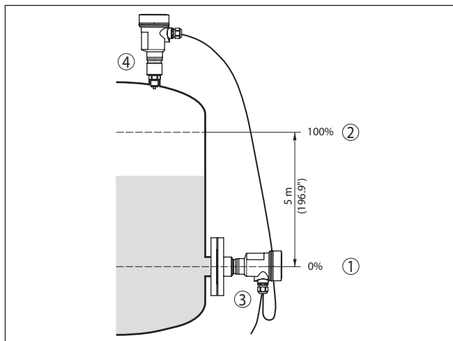
Rys. 23: Przykład parametrów do kompensacji min./max. pomiaru poziomu napętnienia
