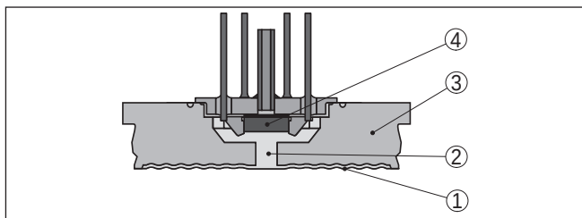
Rys. 2: Budowa układu pomiarowego z czujnikiem piezorezystancyjnym
