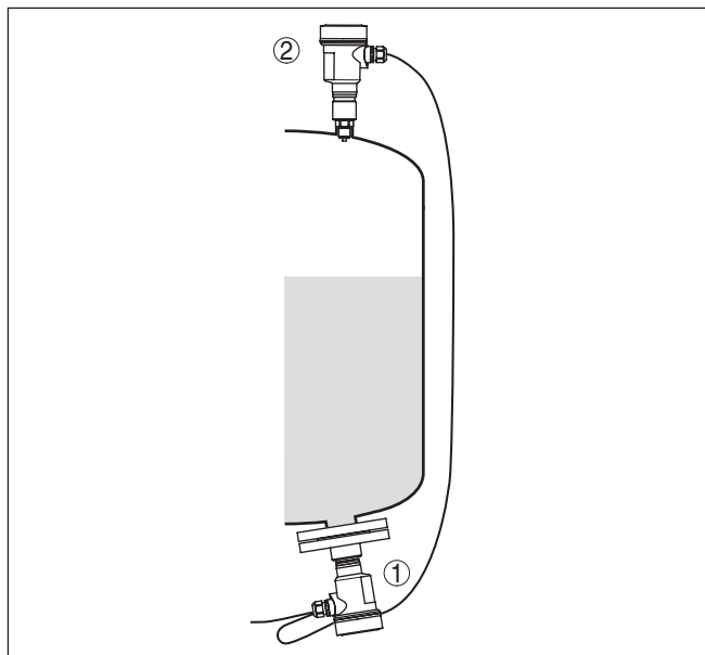
Rys. 10: Rozmieszczenie miejsc pomiaru przy pomiarze poziomu napęnlania w zbiorniku, w którym występuje ciśnienie
