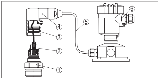
Rys. 24: VEGABAR 83 w wersji wykonania IP68 25 bar z bocznym wylotem kabla, obudowa peryferyjna
