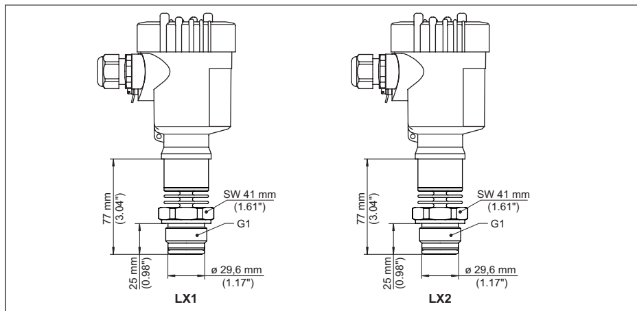
Rys. 39: VEGABAR 83, gwint dla adaptera higienicznego
