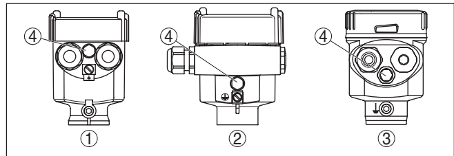
Abb. 2: Position des Filterelementes - Nicht-Ex- und Ex-ia-Ausführung
