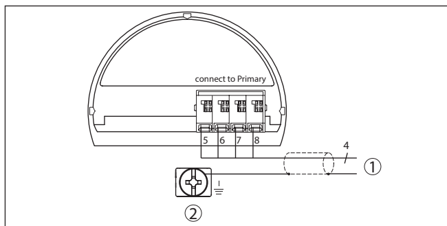
Fig. 4: Aansluitschema VEGABAR 81 secondary device
