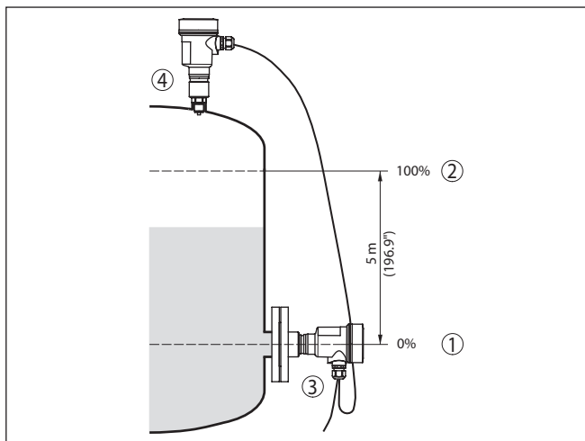
Fig. 8: Parametrevoorbeeld min.-/max.-inregeling niveaumeting
