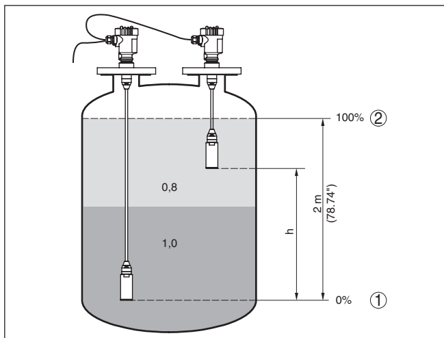
Abb. 8: Parametrierbeispiel Min.-/Max.-Abgleich Trennschichtmessung
