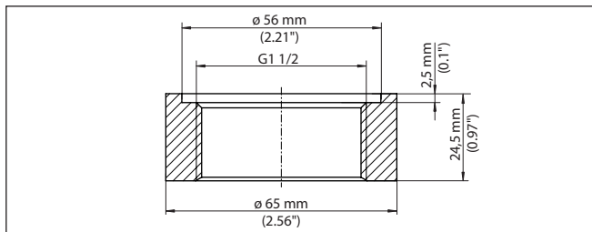
Fig. 23: Dimensions of welded socket, thread G1½ (EN 837) - VEGABAR 82, 83, 86, 87
