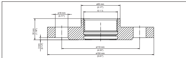
Fig. 36: Dimensions of threaded adapter G1½ (DIN 3852-X) on flange DN 40 (EN 1092-1, Form B1) PN 40
