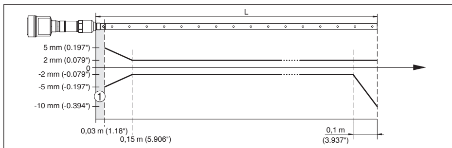
Abb. 31: Messabweichung VEGAFLEX 86 in Koaxialausführung in Medium Wasser (Messlänge bis 1,5 m/4.92 ft)
