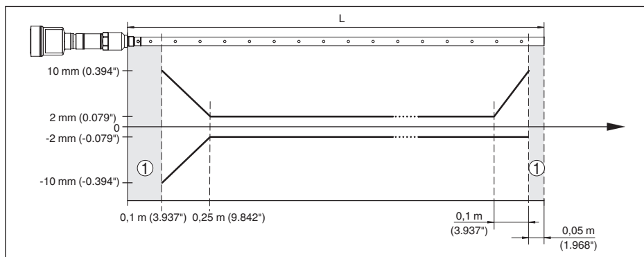
Abb. 33: Messabweichung VEGAFLEX 86 in Koaxialausführung in Medium Öl (Messlänge bis 1,5 m/4.92 ft)
