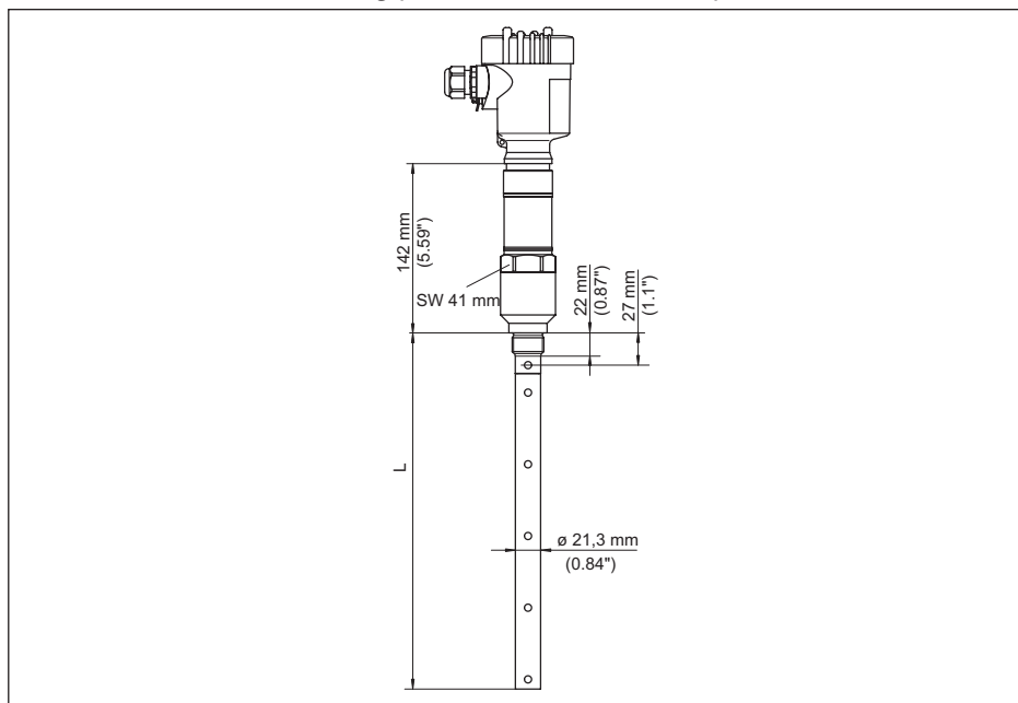
Abb. 41: VEGAFLEX 86, Koaxialausführung mit Gewinde (-20 ... +250 °C/-4 ... +482 °F)
