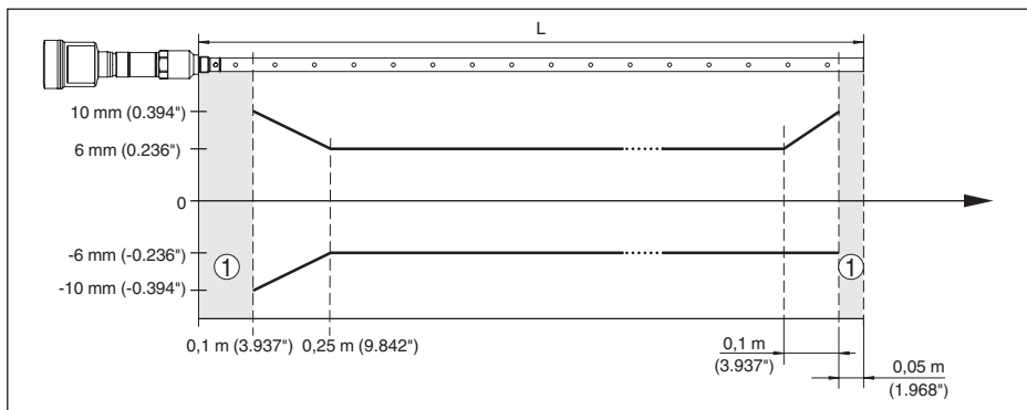
Abb. 34: Messabweichung VEGAFLEX 86 in Koaxialausführung in Medium Öl (Messlänge bis 6 m/19.69 ft)
