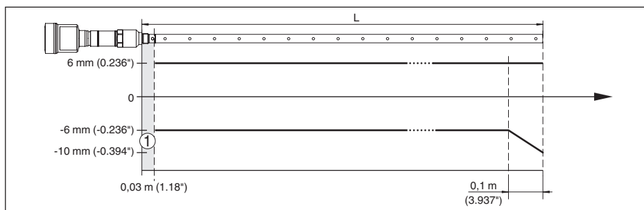
Abb. 32: Messabweichung VEGAFLEX 86 in Koaxialausführung in Medium Wasser (Messlänge bis 6 m/19.69 ft)
