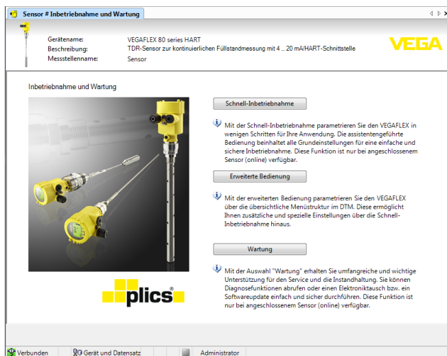
Abb. 27: Schnellinbetriebnahme auswählen
