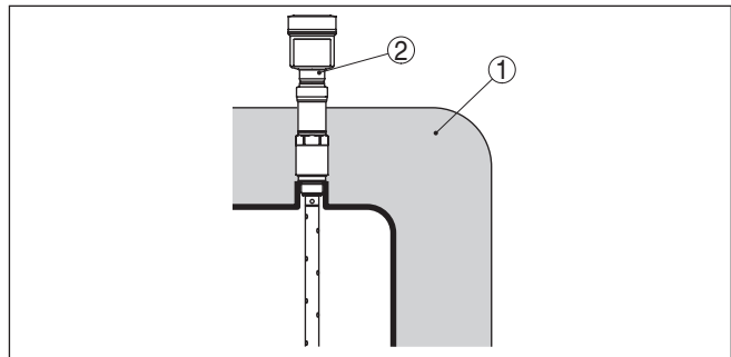
Abb. 7: Montage des Gerätes bei isolierten Behältern.
