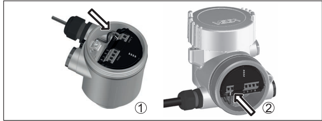
Abb. 9: Anschlussschritte 5 und 6
