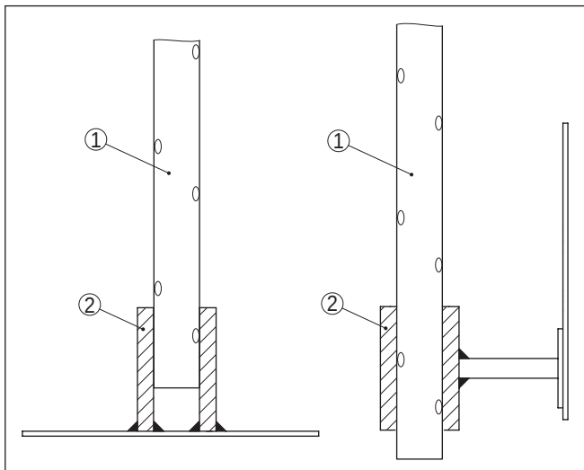
Abb. 8: Messsonde fixieren
