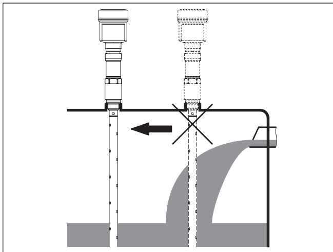
Abb. 5: Montage des Sensors bei einströmendem Medium
