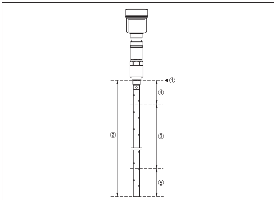
Abb. 30: Messbereiche - VEGAFLEX 86
