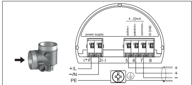
Fig. 9: Compartiment de raccordement boîtier deux chambres pour tension de réseau
