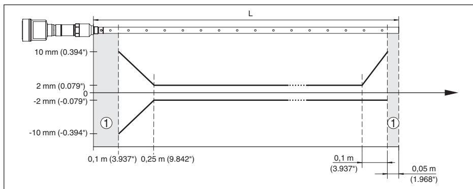
Fig. 28: Écart de mesure VEGAFLEX 86 en version coaxiale dans l'huile (longueur de mesure jusqu'à 1,5 m/4.92 ft)
