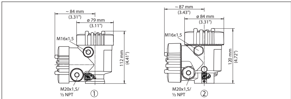
Fig. 31: VEGAFLEX 86 avec module de réglage et d'affichage intégré, la hauteur du boîtier augmente de 9 mm (0,35 in)
