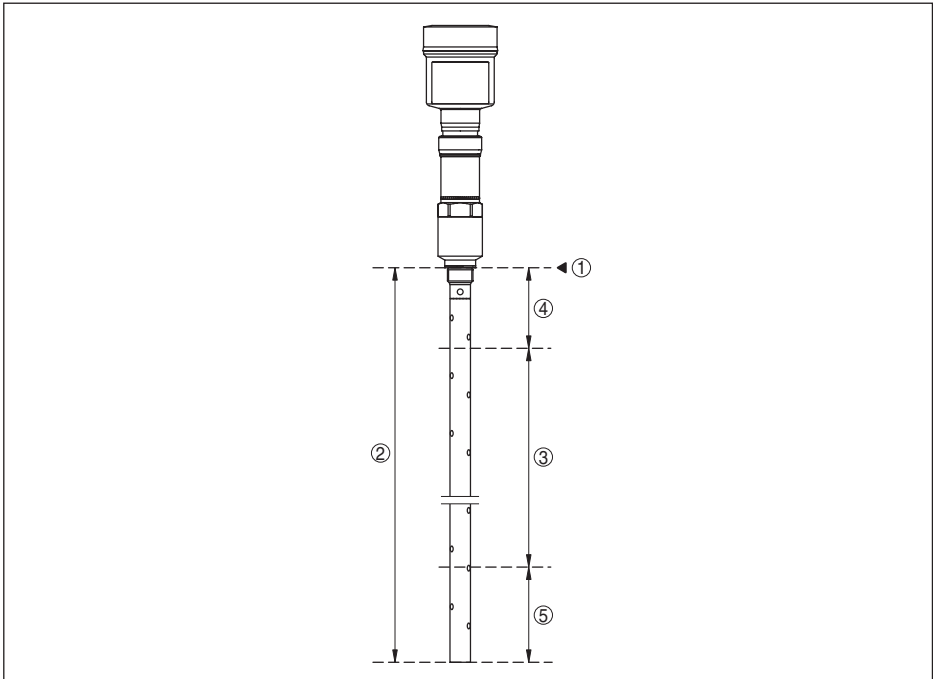
Fig. 25: Plages de mesure - VEGAFLEX 86
