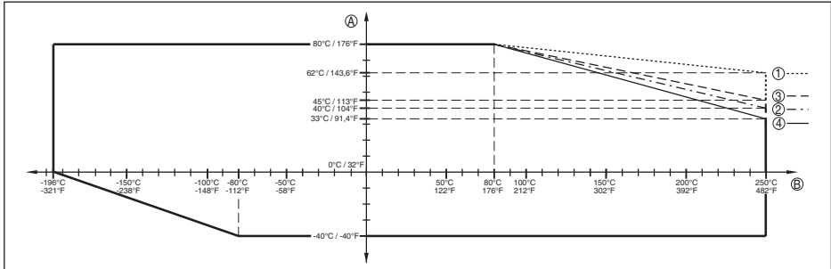
Fig. 30: Température ambiante - température process, version standard
