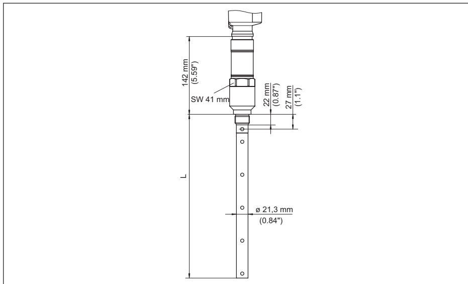
Fig. 32: VEGAFLEX 86 - version coaxiale avec filetage (-20 ... +250 °C/-4 ... +482 °F)
