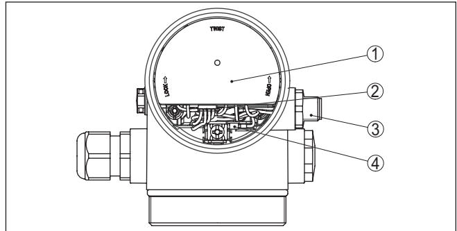
Fig. 11: Vue sur le compartiment de l'électronique avec l'adaptateur VEGADIS pour le raccordement de l'unité de réglage et d'affichage
