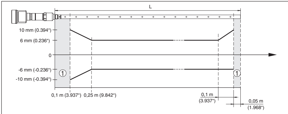
Fig. 29: Écart de mesure VEGAFLEX 86 en version coaxiale dans l'huile (longueur de mesure jusqu'à 6 m/19.69 ft)
