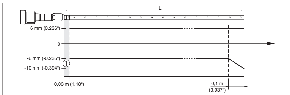
Fig. 27: Écart de mesure VEGAFLEX 86 en version coaxiale dans l'eau (longueur de mesure jusqu'à 6 m/19.69 ft)
