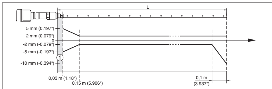
Fig. 26: Écart de mesure VEGAFLEX 86 en version coaxiale dans l'eau (longueur de mesure jusqu'à 1,5 m/4.92 ft)
