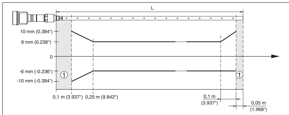
Fig. 31: Meetafwijking VEGAFLEX 86 in coaxuitvoering in medium olie (meetlengte tot 6 m/19.69 ft)
