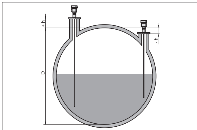
Fig. 21: Tankhoogte en sokcorrectiewaarde
