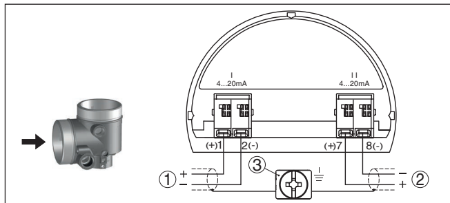
Fig. 17: Aansluitruimte tweekamerbehuizing, extra elektronica - extra stroomuitgang
