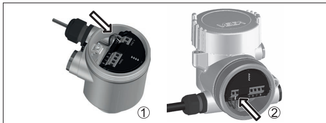
Fig. 8: Aansluitstappen 5 en 6
