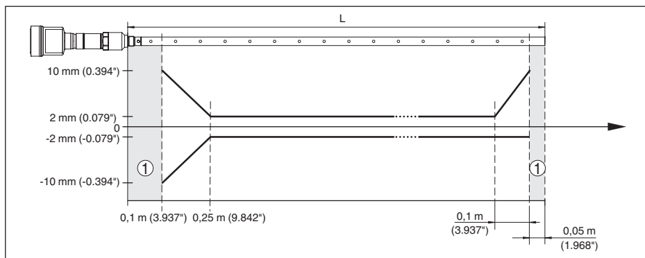
Fig. 30: Meetafwijking VEGAFLEX 86 in coaxuitvoering in product olie (meetlengte tot 1,5 m/4.92 ft)
