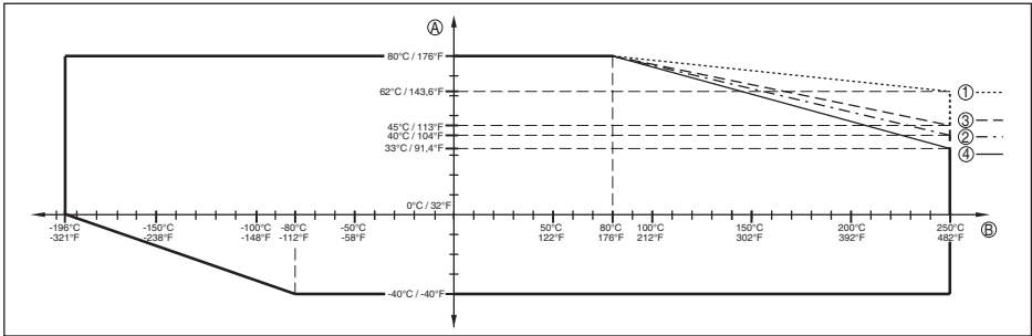
Fig. 32: Omgevingstemperatuur - procestemperatuur standaarduitvoering
