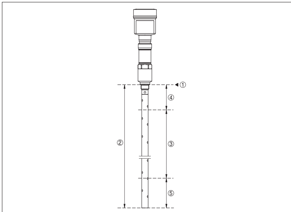
Fig. 27: Meetbereiken - VEGAFLEX 86
