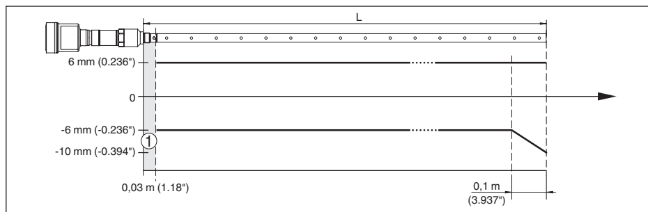
Fig. 29: Meetafwijking VEGAFLEX 86 in coaxuitvoering in product water (meetlengte tot 6 m/19.69 ft)
