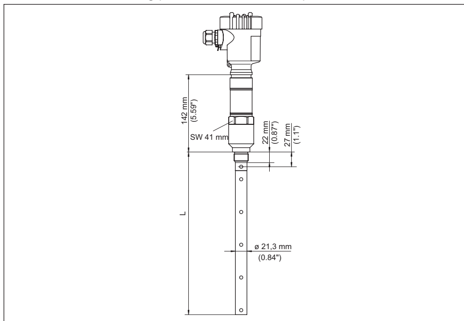
Fig. 38: VEGAFLEX 86, coaxuitvoering met schroefdraad (-20 ... +250 °C/-4 ... +482 °F)
