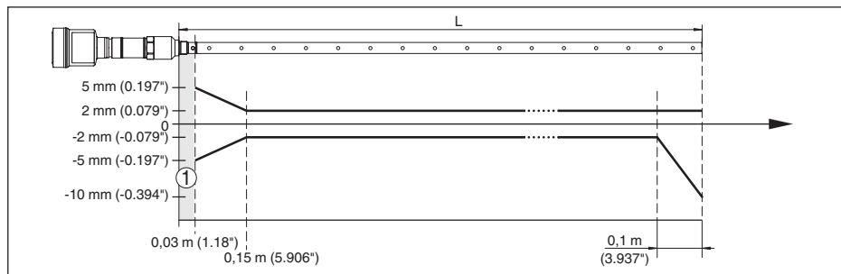
Fig. 28: Meetafwijking VEGAFLEX 86 in coaxuitvoering in product water (meetlengte tot 1,5 m/4.92 ft)
