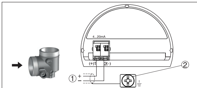
Fig. 20: Aansluitruimte - Ex-d-ia-tweekamerbehuizing
