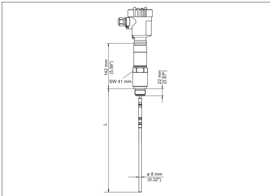
Fig. 51: VEGAFLEX 86, schroefdraaduitvoering
