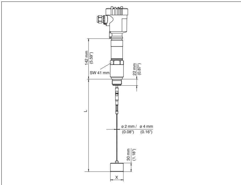
Fig. 50: VEGAFLEX 86, schroefdraaduitvoering met centreergewicht
