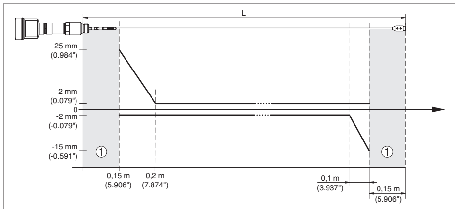
Fig. 42: Meetafwijking VEGAFLEX 86 in kabeluitvoering (4 mm/0.157 in), in medium olie
