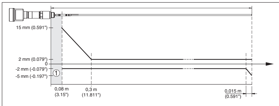
Fig. 38: Meetnauwkeurigheid VEGAFLEX 86 in staafuitvoering in medium water
