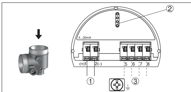
Fig. 19: Elektronicaruimte - Ex-ia-tweekamerbehuizing
