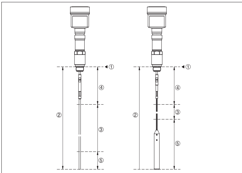
Fig. 37: Meetbereiken - VEGAFLEX 86
