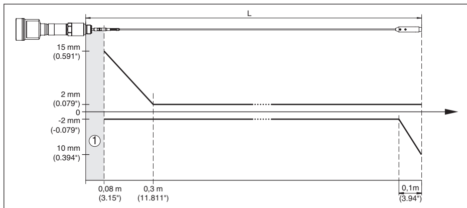
Fig. 40: Meetnauwkeurigheid VEGAFLEX 86 in kabeluitvoering in medium water
