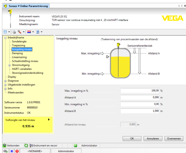
Fig. 31: Voorbeeld van een DTM-aanzicht
