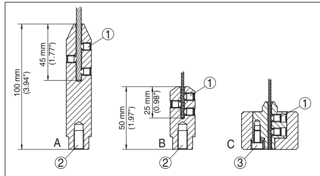
Fig. 36: Kabelmeetsonde inkorten
