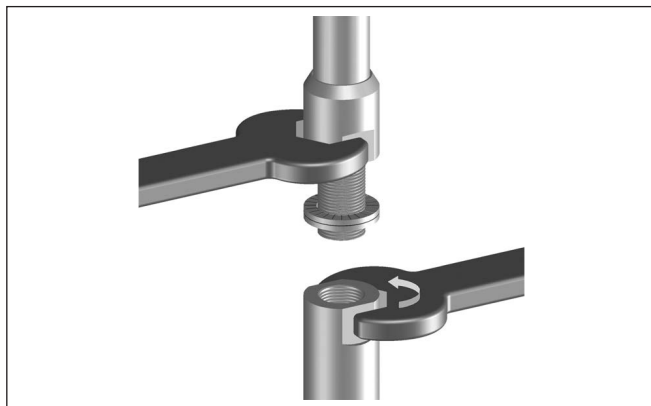
Fig. 35: Meetkabel resp. meetstaaf vervangen
