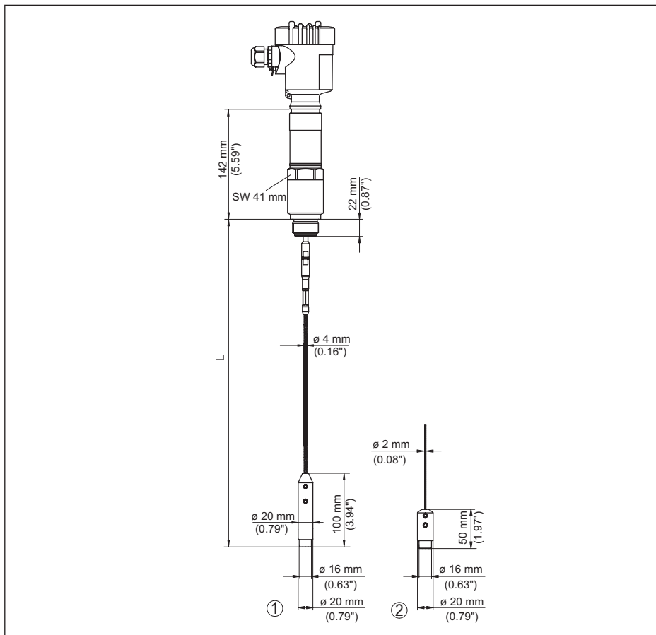
Fig. 49: VEGAFLEX 86, schroefdraaduitvoering met spangewicht (alle spangewichten met schroefdraad M8 voor oogbout)
