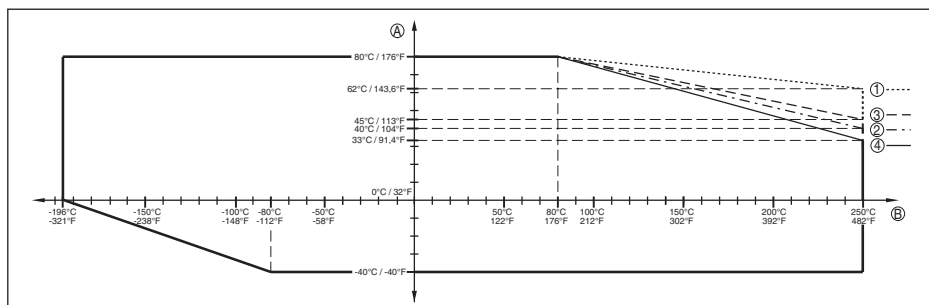
Fig. 43: Omgevingstemperatuur - procestemperatuur standaarduitvoering
