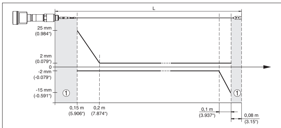
Fig. 41: Meetafwijking VEGAFLEX 86 in kabeluitvoering (2 mm/0.079 in), in medium olie
