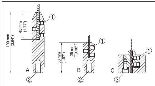
Fig. 36: Kabelmeetsonde inkorten
