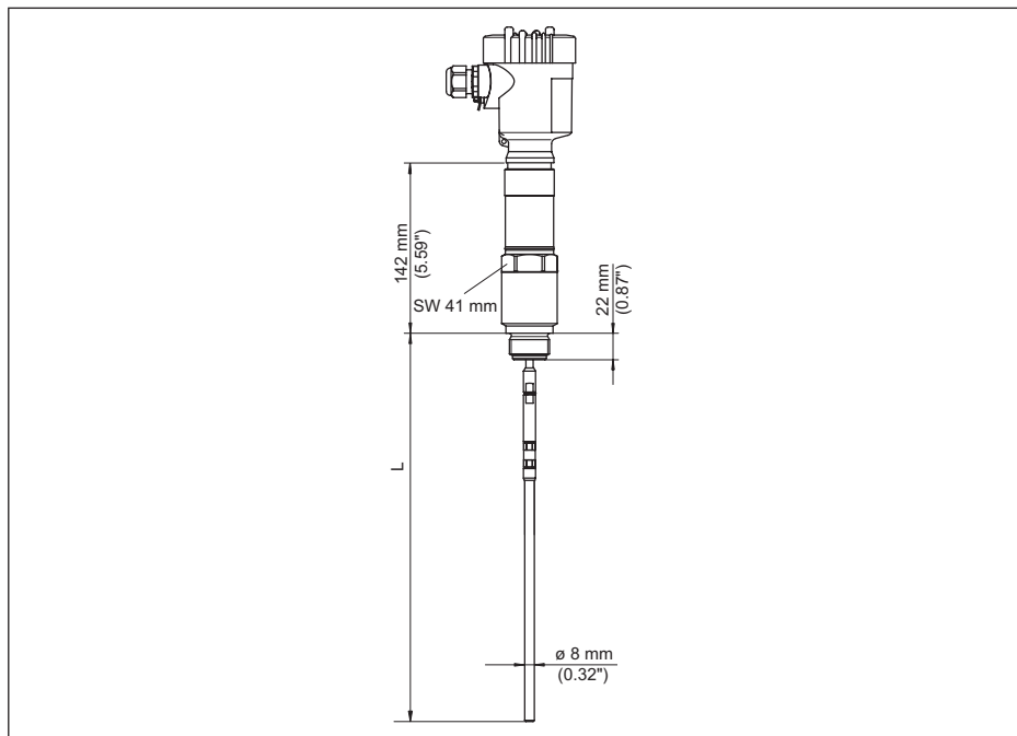
Fig. 51: VEGAFLEX 86, schroefdraaduitvoering
