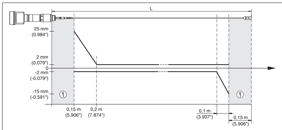
Fig. 42: Meetafwijking VEGAFLEX 86 in kabeluitvoering (4 mm/0.157 in), in medium olie
