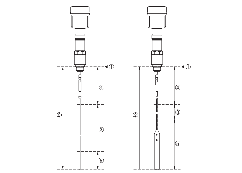
Fig. 37: Meetbereiken - VEGAFLEX 86
