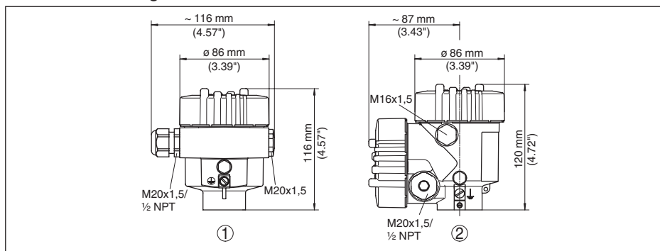
Fig. 45: Huisuitvoeringen in beschermingsklasse IP66/IP68 (0,2 bar), (met ingebouwde display- en bedieningsmodule wordt het huis 9 mm/0.35 in hoger)
