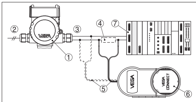
Fig. 24: Aansluiting van de PC via HART op de signaalkabel
