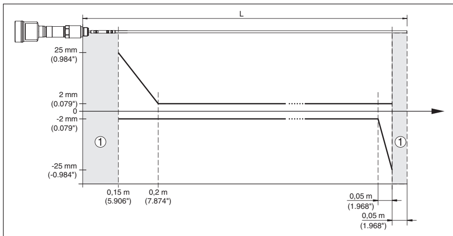
Fig. 33: Meetnauwkeurigheid VEGAFLEX 86 in staafuitvoering in medium olie
