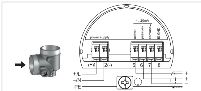
Fig. 16: Aansluitruimte tweekamerbehuizing bij netspanning
