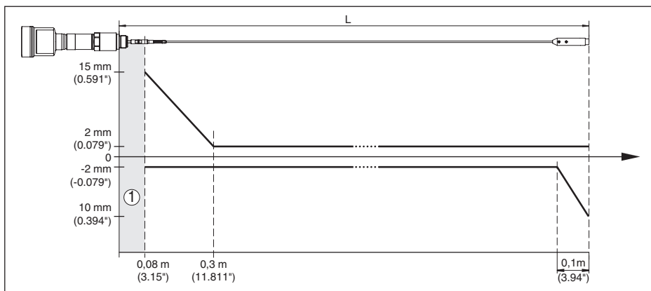
Fig. 34: Meetnauwkeurigheid VEGAFLEX 86 in kabeluitvoering in medium water
