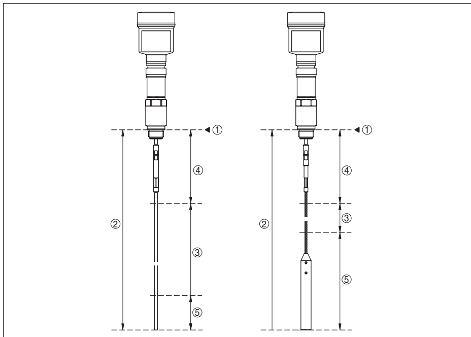
Fig. 31: Meetbereiken - VEGAFLEX 86
