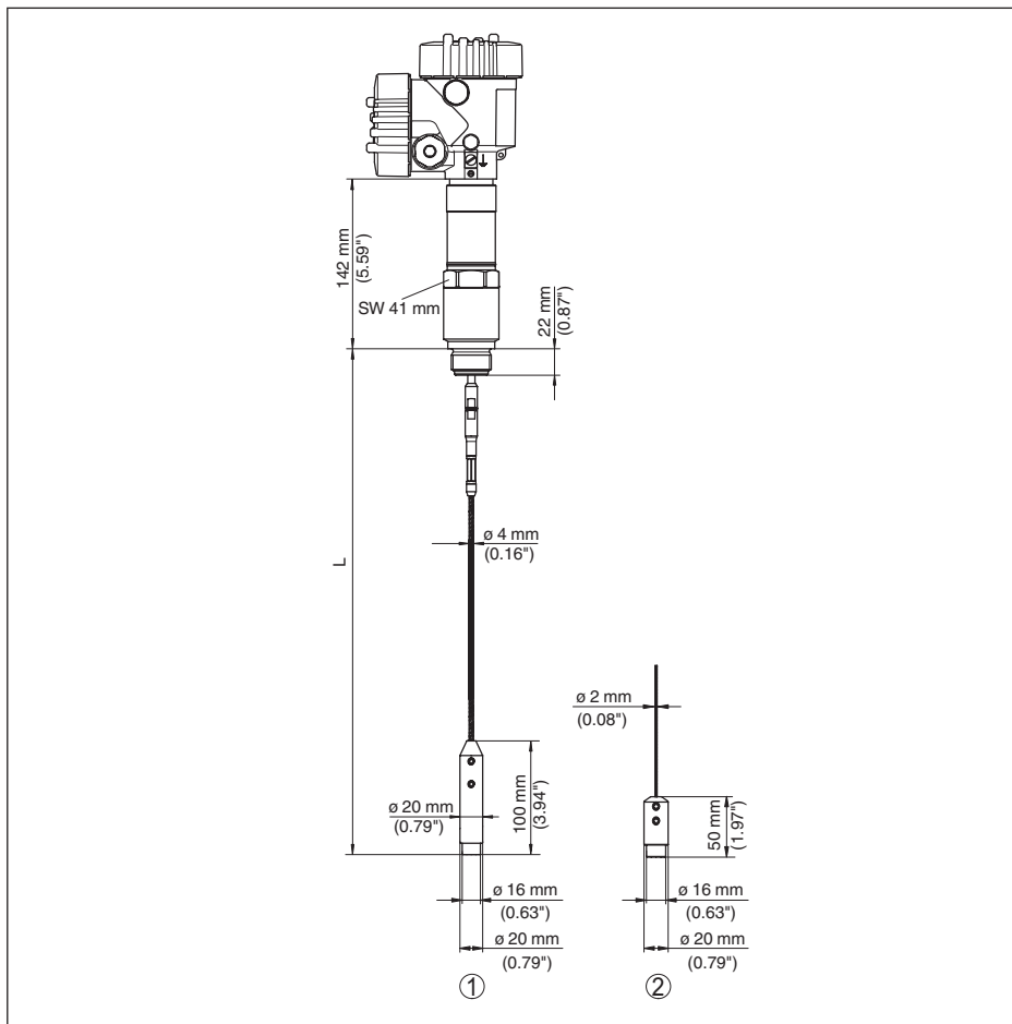
Fig. 39: VEGAFLEX 86, schroefdraaduitvoering met spangewicht (alle spangewichten met schroefdraad M8 voor oogbout)
