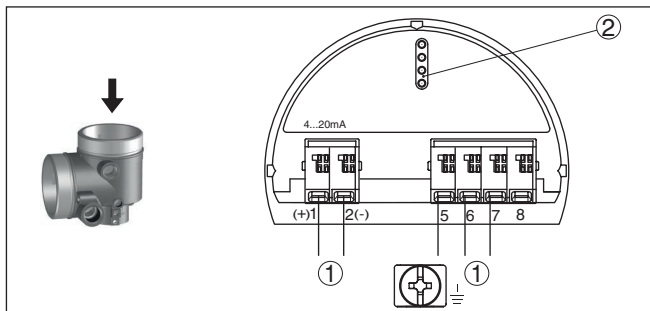
Fig. 15: Elektronicaruimte - tweekamerbehuizing
