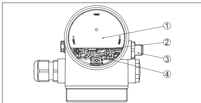
Fig. 18: Een blik op de elektronicarimte met VEGADIS-adapter voor aansluiting van de externe display- en bedieningseenheid
