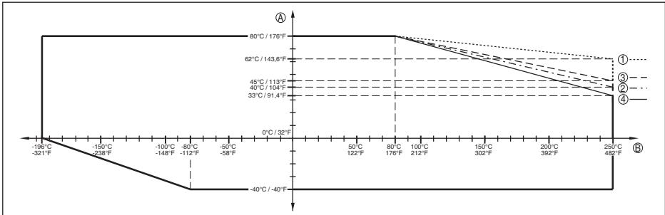
Fig. 37: Omgevingstemperatuur - procestemperatuur standaarduitvoering
