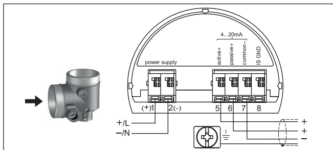
Fig. 17: Aansluitruimte tweekamerbehuizing bij laagspanning
