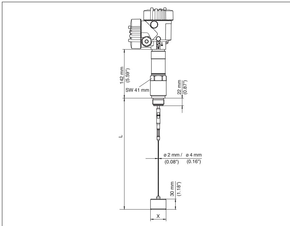
Fig. 40: VEGAFLEX 86, schroefdraaduitvoering met centreergewicht
