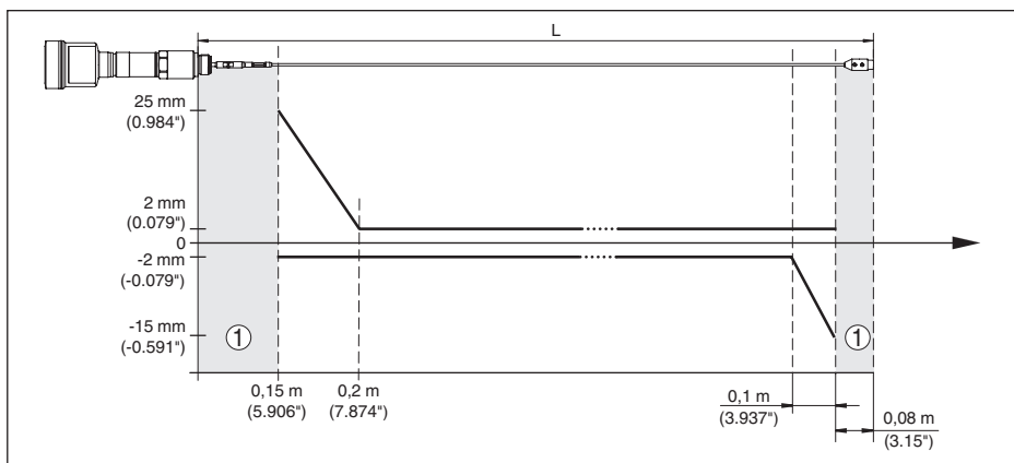
Fig. 35: Meetafwijking VEGAFLEX 86 in kabeluitvoering (2 mm/0.079 in), in medium olie
