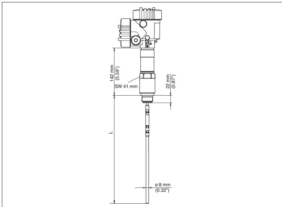
Fig. 41: VEGAFLEX 86, schroefdraaduitvoering
