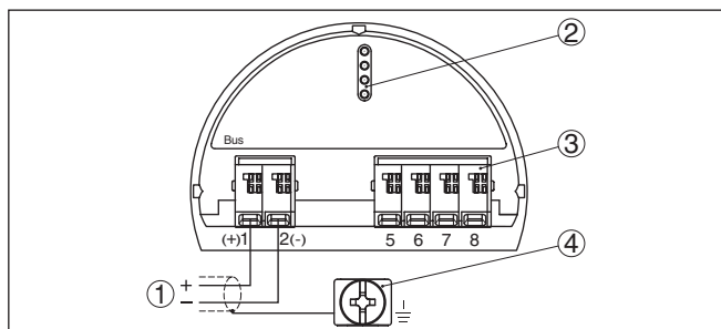
Fig. 8: Aansluitruimte - tweekamerbehuizing
