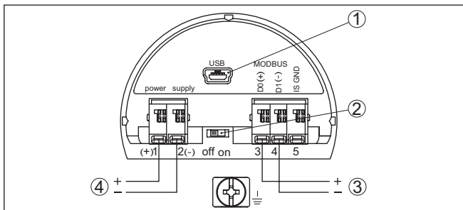
Abb. 8: Anschlussraum
